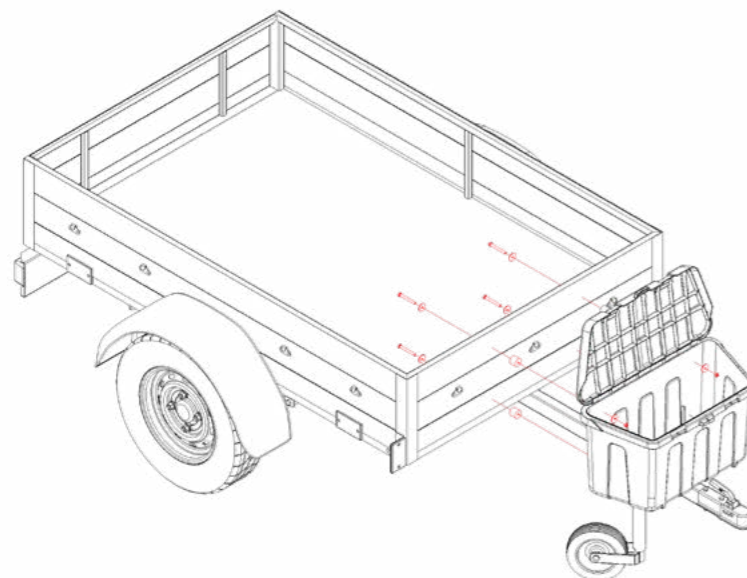
Beispiel für die Montage der Profibox Plus mit dem Montageset.
