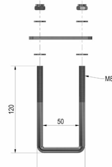
Mit diesem Montageset ist es möglich eine Box auf einer Zugdeichsel zu montieren.
